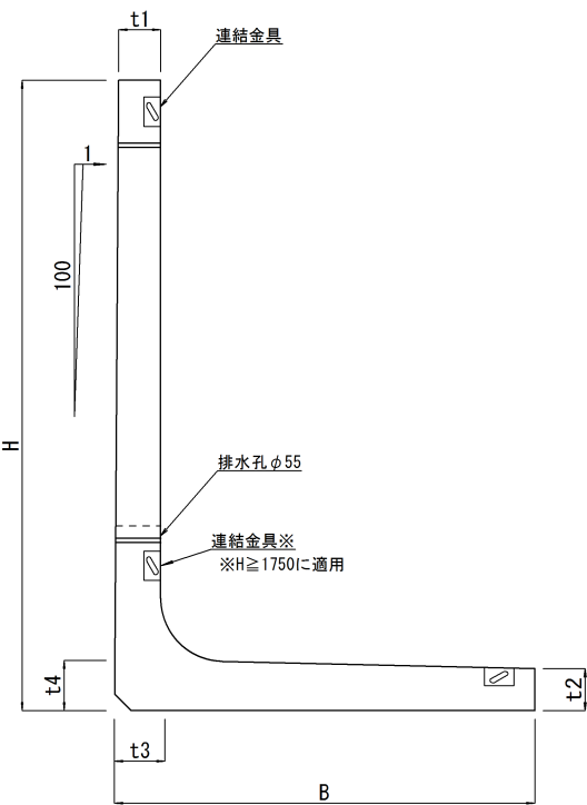
断 面 図
