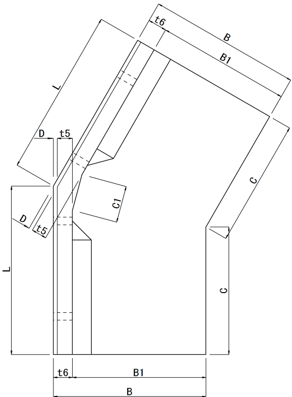
コーナー角度 150° 用
