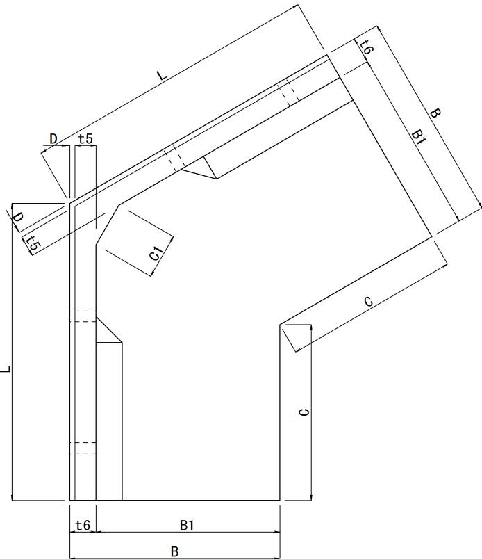
コーナー角度 120° 用
